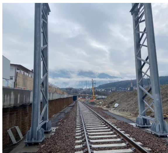
Bild 4: RI31 e TR31 – Absenkung Gleiskörper
