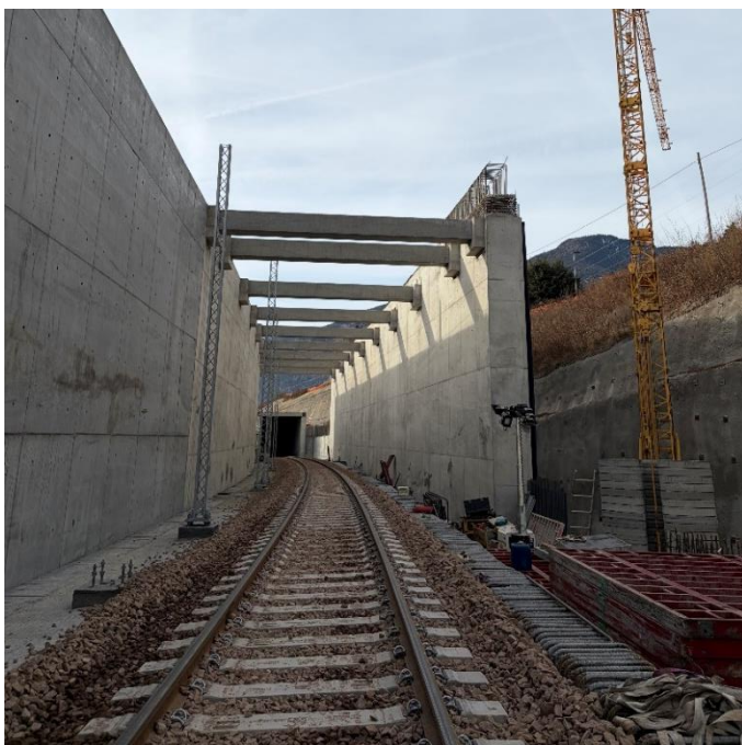
Figura 6: FV01 – Muri laterali
