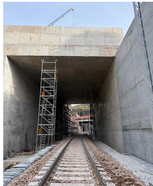
Bild 7: GA07 – Fertigstellung des Tunnels in offener Bauweise
